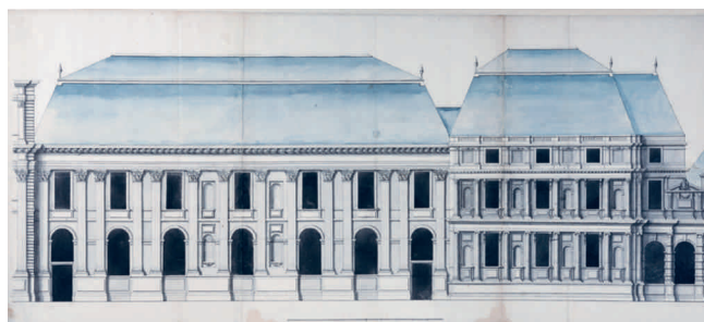
François d'Orbay (1634-1697), Élévation du pavillon et de l'aile de la salle des Machines sur le jardin, 1659 , plume, encre noire et lavis, 43,5 × 99,5 cm, Stockholm, Nationalmuseum, CC 5.
