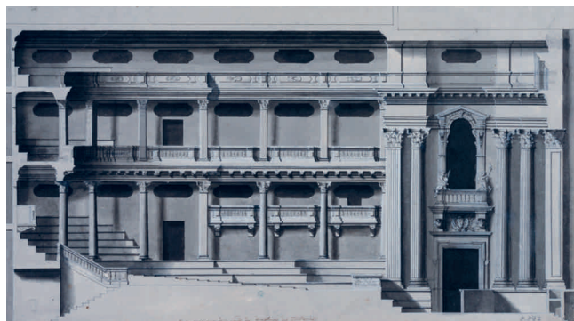
Anonyme, Coupe longitudinale de la salle des Machines, fin du XVII e siècle ? , plume, encre et aquarelle, 22,5 × 41,4 cm, Stockholm, Nationalmuseum, THC 8893.
